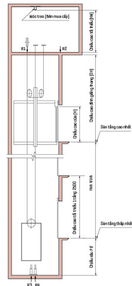
Mặt Cắt đứng giếng thang
