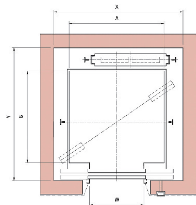
Mặt Cắt Ngang Giếng Thang Đối Trọng Sau
