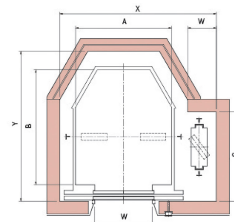
Mặt Cắt ngang giếng thang hình bán lục lăng
