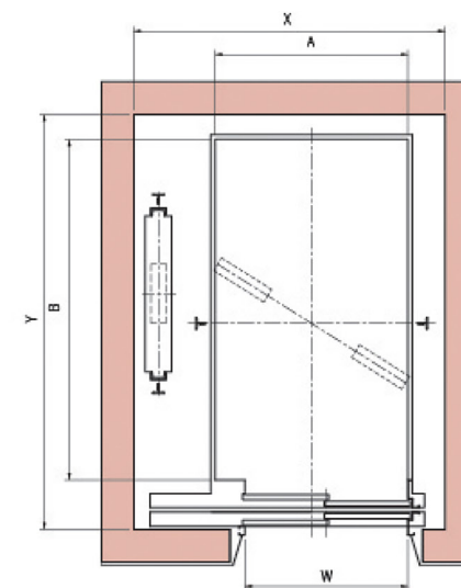
Mặt Cắt ngang giếng thang
