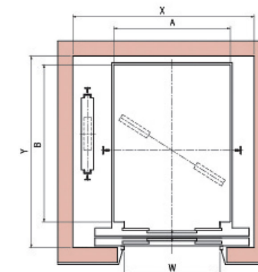
Mặt Cắt ngang giếng thang LOẠI CỬA 2 CỎ
