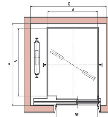
Loại cửa 2S
