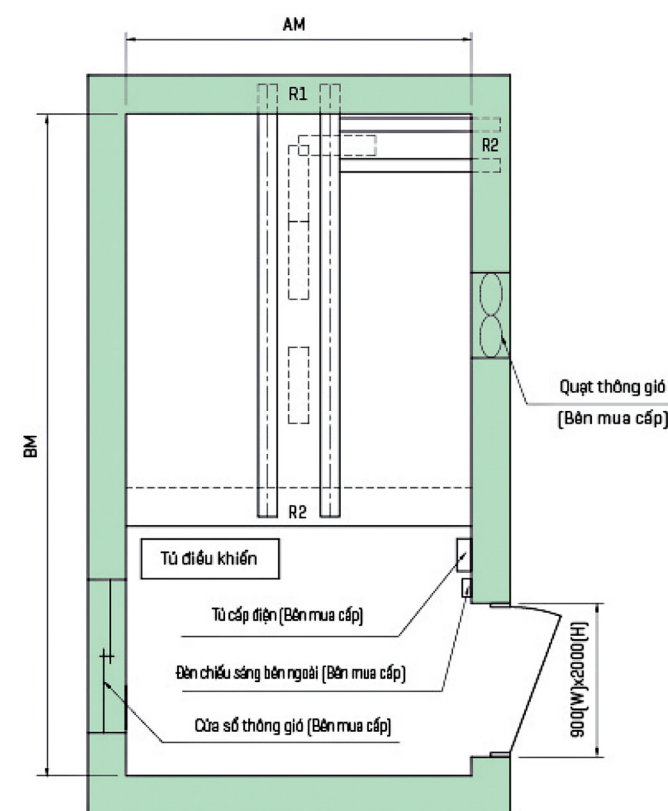
Mặt cắt ngang phòng máy
