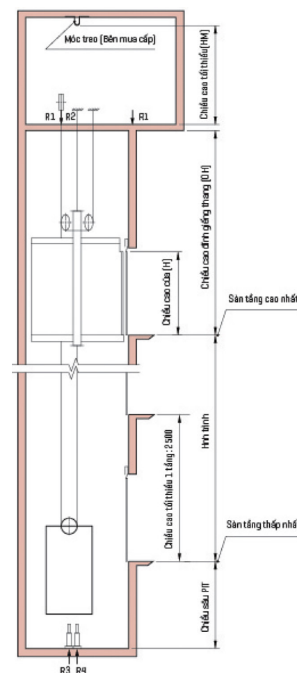
Mặt Cắt đứng giếng thang
