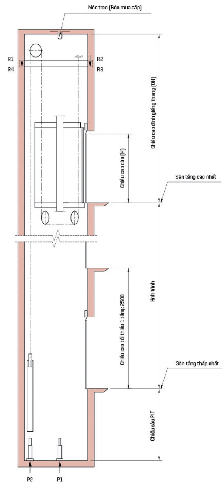
Đối trọng bên
