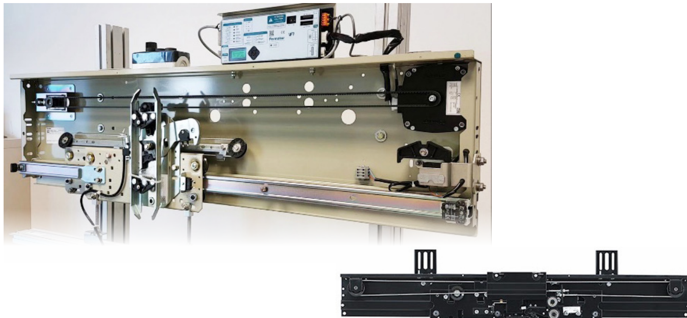
BỘ CHUYỂN ĐỘNG CỬA CABIN & TẦNG (CHINA,KOREA)
