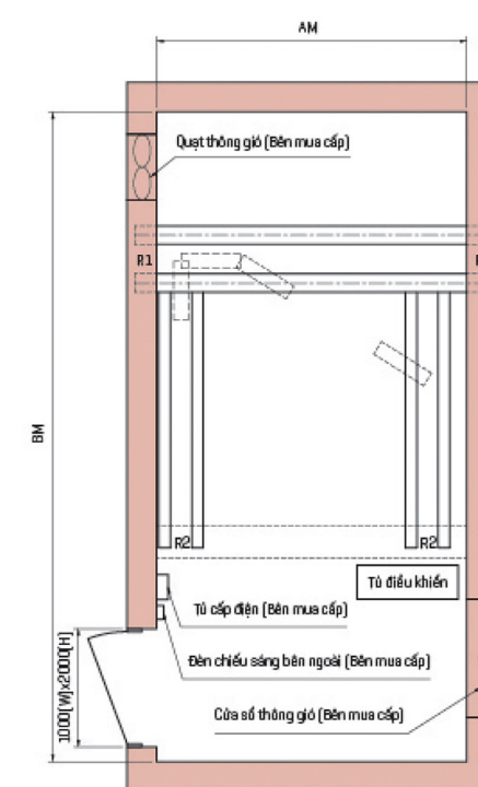
Mặt Cắt ngang phòng máy
