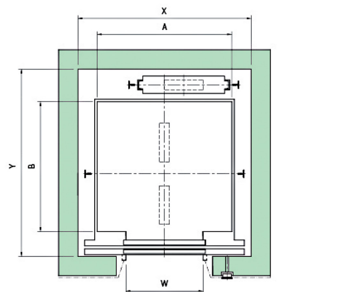
Mặt Cắt Ngang Giếng Thang Đối Trọng Sau
